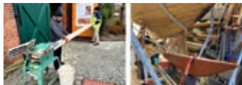
Der provisorische Kielbalken wird auf Maß gehobelt
