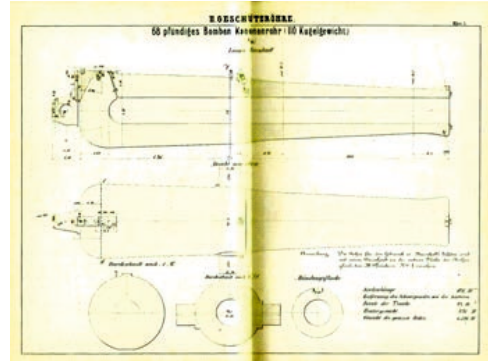
Kanonenrohr einer 68-Pfünder Vorderladerkanone der Preußischen Marine
